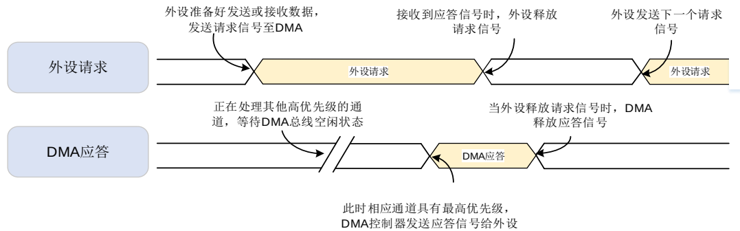
图 10-3. 握手机制
