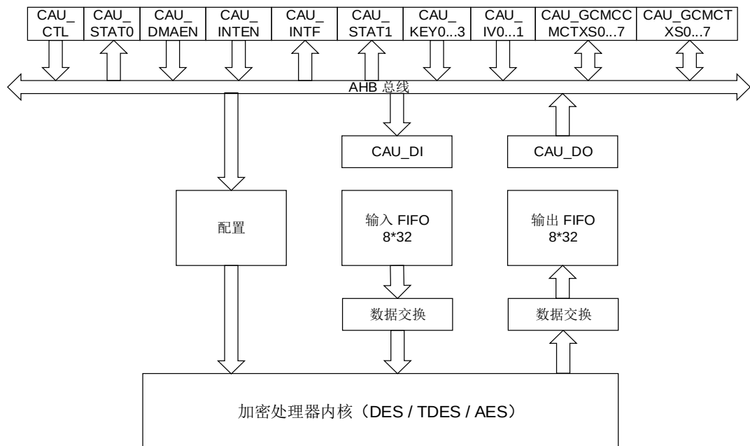
图 20-3. CAU 框图
