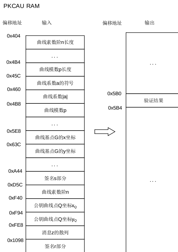
图 22-23. ECDSA 验证
