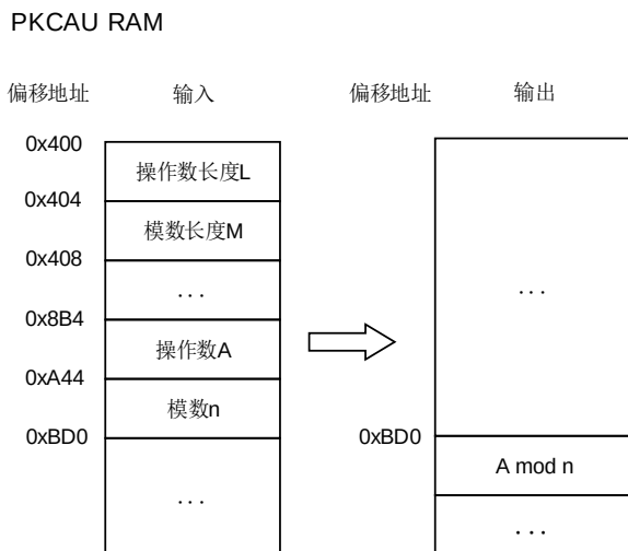
图 22-9. 取模运算
