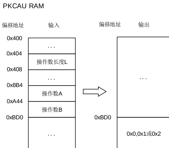
图 22-8. 算术比较
