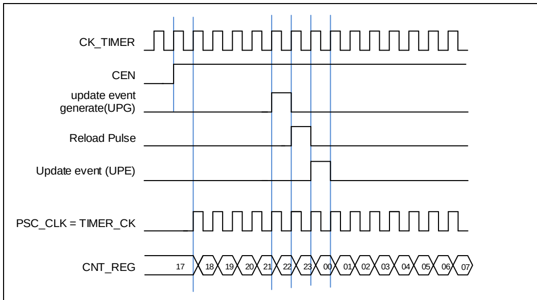
图 15-34. 内部时钟分频为 1 时，计数器的时序图
