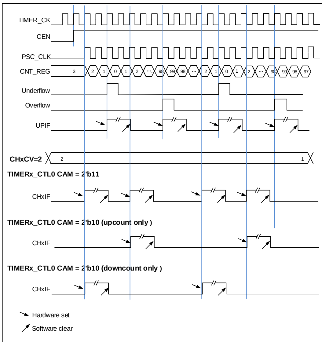
图 15-8. 中央计数模式计数器时序图
