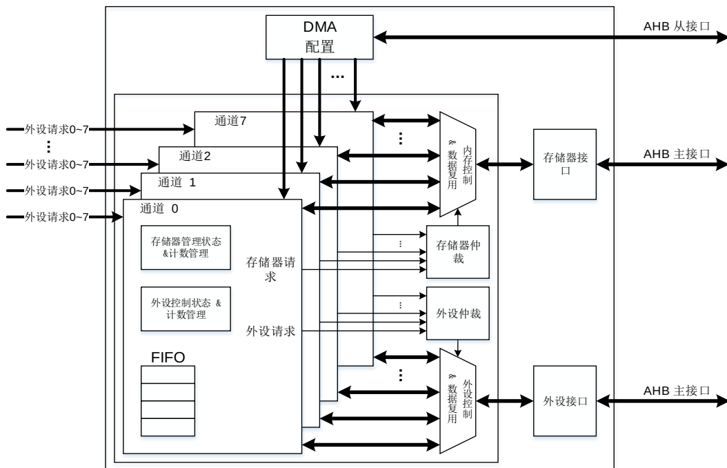
图 10-1. 系统架构
