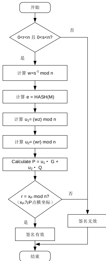
图 22-4. ECDSA 验证流程图
