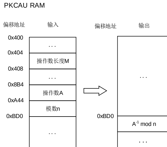
图 22-17. 模逆运算
