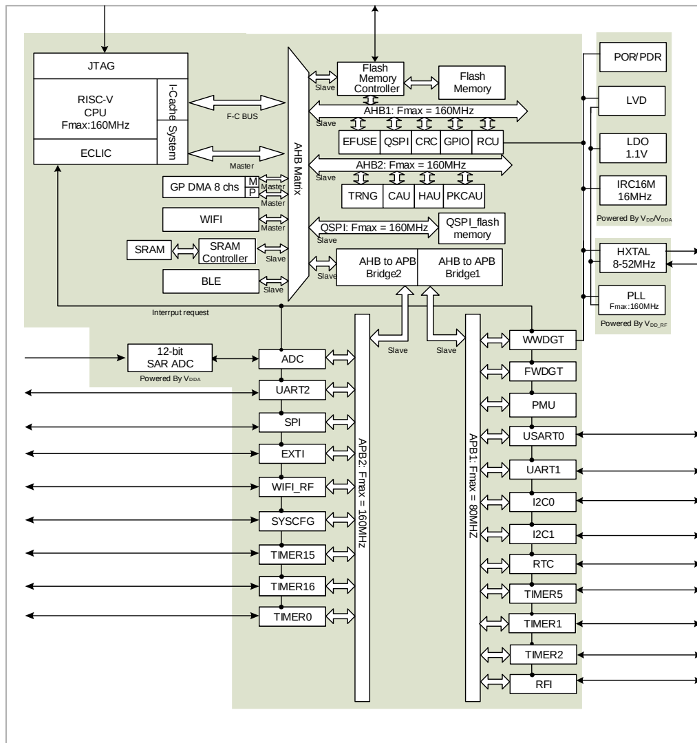
图 1-1. GD32VW55x 系列器件的系统架构示意图
